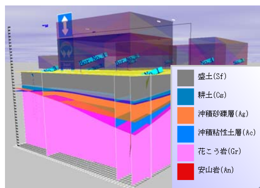
図-2 学校敷地の3次元地質モデルデータ
