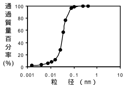
図-2 噴砂の粒径加積曲線
